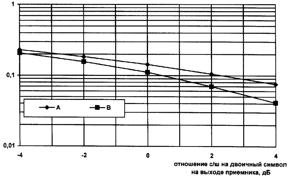
Вероятность ошибки до декодера Витерби
